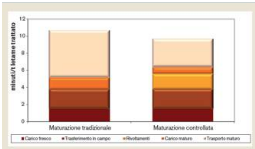
● Gráfico 3 - Tempi di lavorazione meccanica
